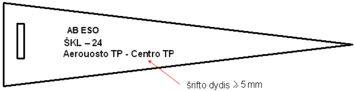
61 pav. Ryšių kabelių žymėjimo švininė juostelė, tvirtinimui tiesiai ant \geq 32 mm skersmens vamzdelių
