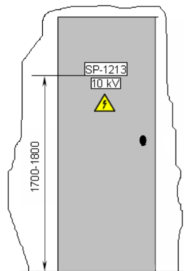
7 pav. 10 kV skirstomojo punkto 10 kV skirstyklos durų žymenys
