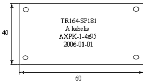
51 pav. 0,4 kV kabelio žymuo trasoje
