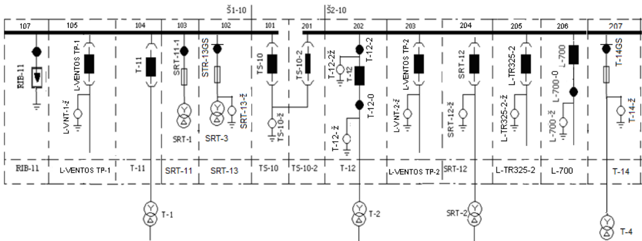
a) Naujai sumontuoto ar rekonstruoto (po atlikto „retrofito“) skirstomojo punkto žymenys
