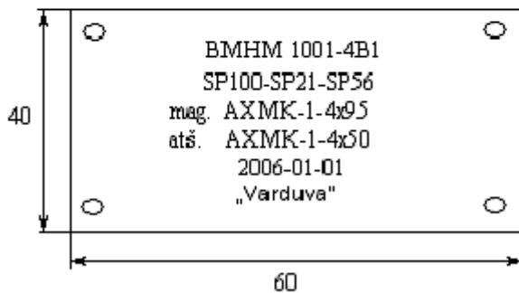
53 pav. 0,4 kV atšakinės movos žymuo
