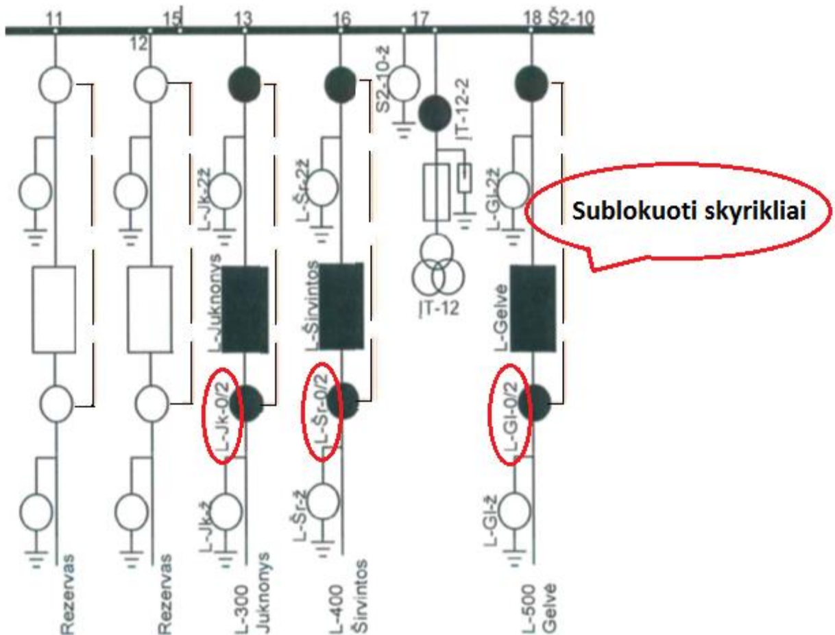
26 c) pav. 10 kV seno KSO ir/ar KRU tipo narveliuose sublokuotų (šyningo ir linijinio) skyriklių žymėjimas.
