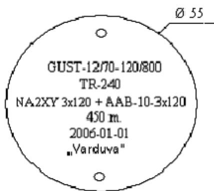
A 45 pav. 10 kV galinės movos žymuo, A esant papildomai prijungtam kabeliui, žymuo B be papildomai prijungto kabelio
