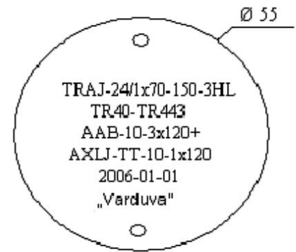
49 pav. 10 kV pereinamosios movos žymuo
