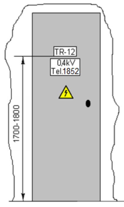
10 pav. Transformatorinės 0,4 kV skirstyklos durų žymenys
