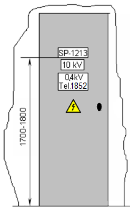
8 pav. 10 kV skirstomojo punkto vienoje patalpoje įrengtų 10 ir 0,4 kV skirstyklų durų žymenys
