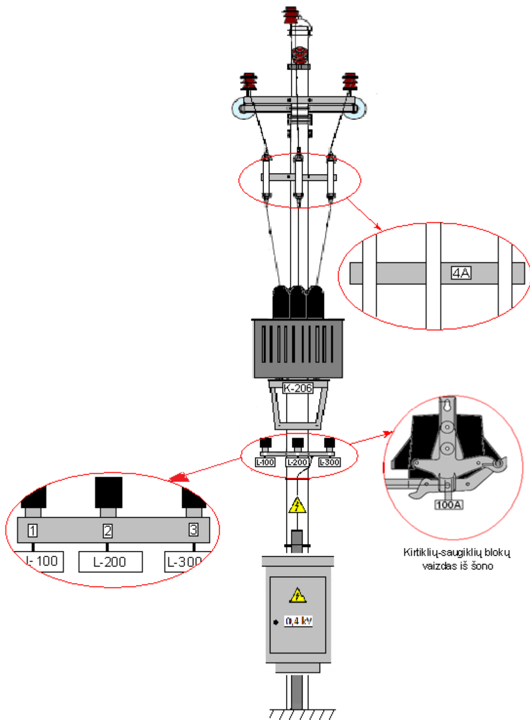
15 pav. Stulpinės transformatorinės žymenys
