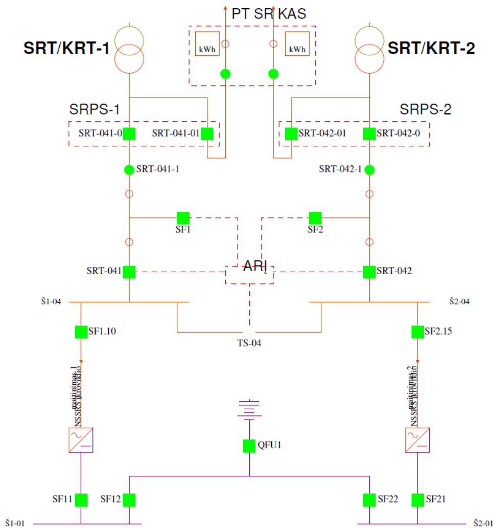
44 pav. Kintamosios srovės savųjų reikiųjų skydo žymenys
