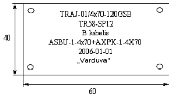
54 pav. 0,4 kV pereinamosios movos žymuo
