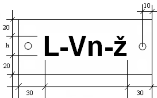
2 pav. Skyriklio arba įžemiklio pavadinimo plokštelė
