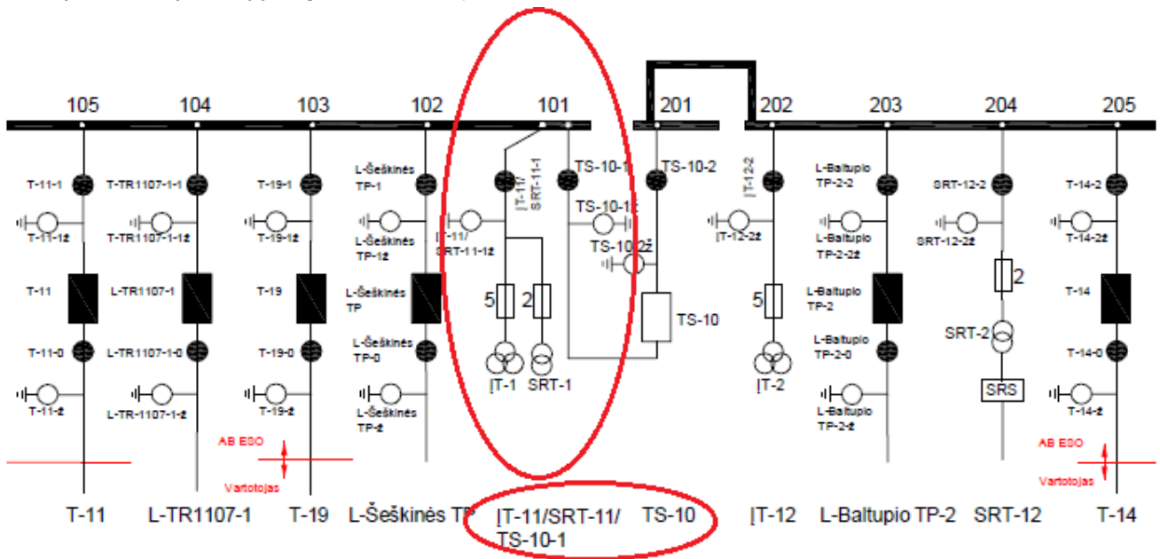
26 b) pav. Kuomet viename narvelyje yra keli technologiniai įrenginiai (savųjų reikmių ir (ar) įtampos transformatoriai ir t. t.)
