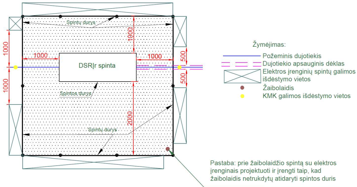
1 paveikslas. Prie DSRĮr aikštelės ribos elektros įrenginių spintų išdėstymas
