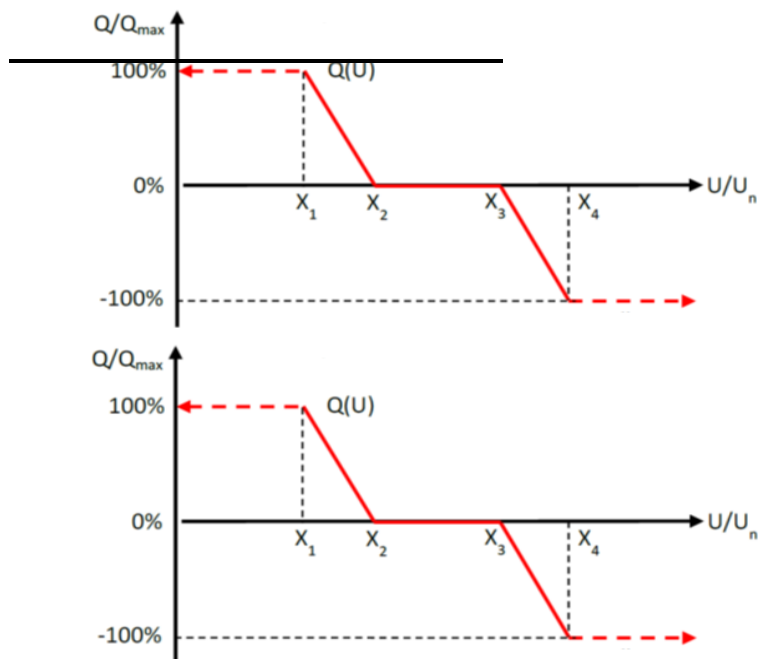
3 paveikslas. Elektros jėgainių parko modulių įtampos ir reaktyviosios galios valdymo Q(U) statinė charakteristika
