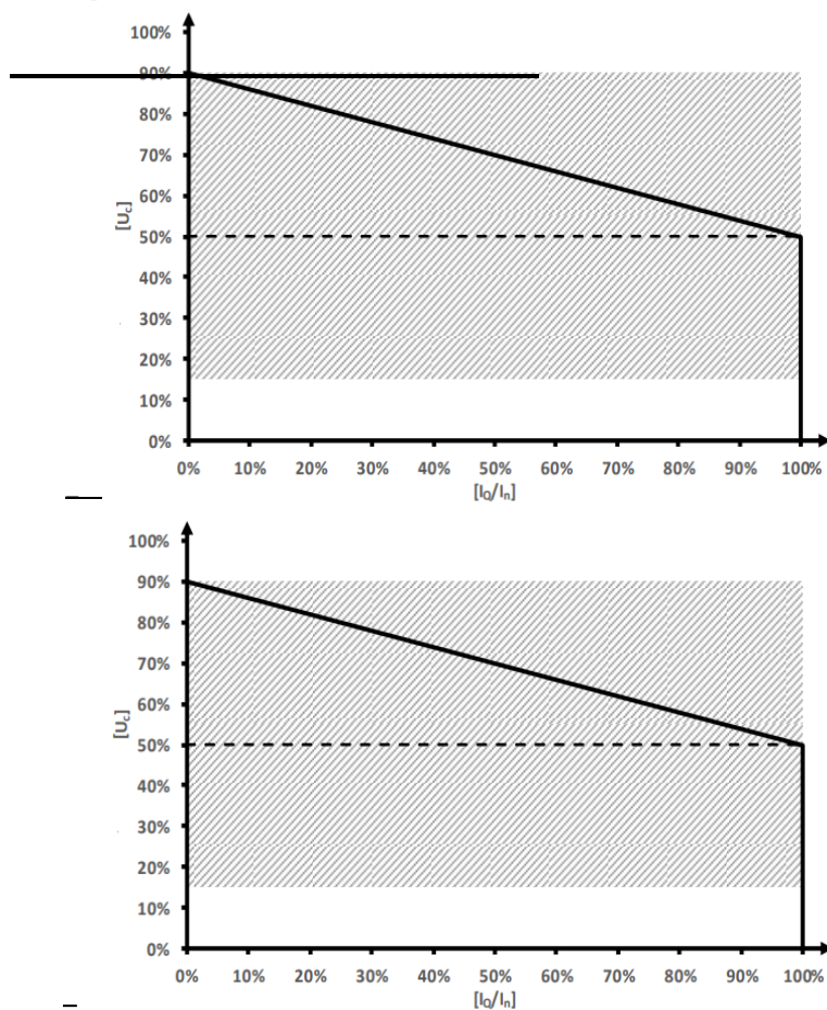
1 paveikslas. Elektros jėgainių parko modulių trikties srovės tiekimo charakteristika
