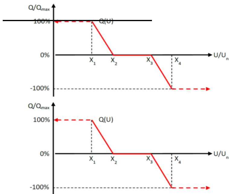
2 paveikslas. Elektros jėgainių parko modulių įtampos ir reaktyviosios galios valdymo Q(U) statinė charakteristika
